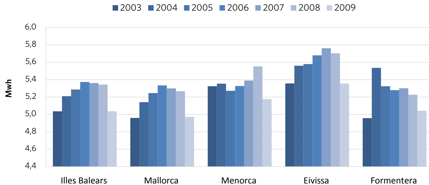
12.14 Evolució del consum elèctric per habitant i any Evolución del consumo eléctrico por habitante y año
