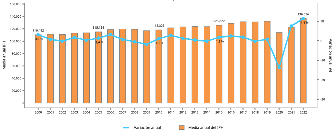
Valores anuales medios del indicador de presión humana en Menorca: 2000-2022
