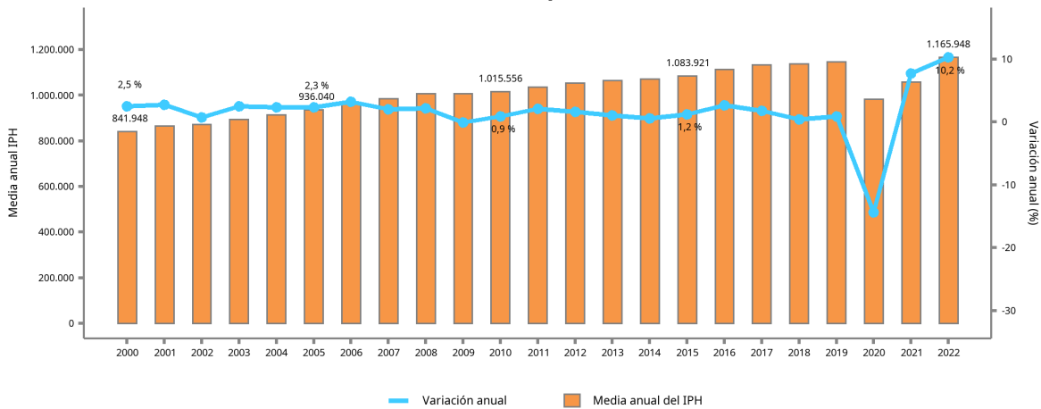
Valores anuales medios del indicador de presión humana en Mallorca: 2000-2022
