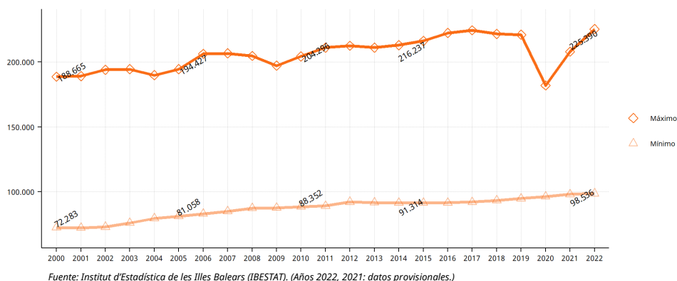
Valores máximos y mínimos anuales del indicador de presión humana en Menorca: 2000-2022
