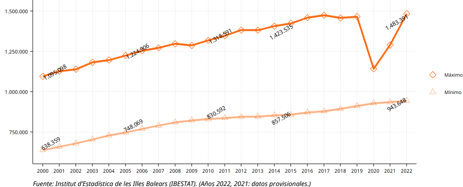
Valores máximos y mínimos anuales del indicador de presión humana en Mallorca: 2000-2022
