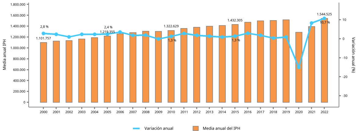
Valores anuales medios del indicador de presión humana en las Illes Balears: 2000-2022
