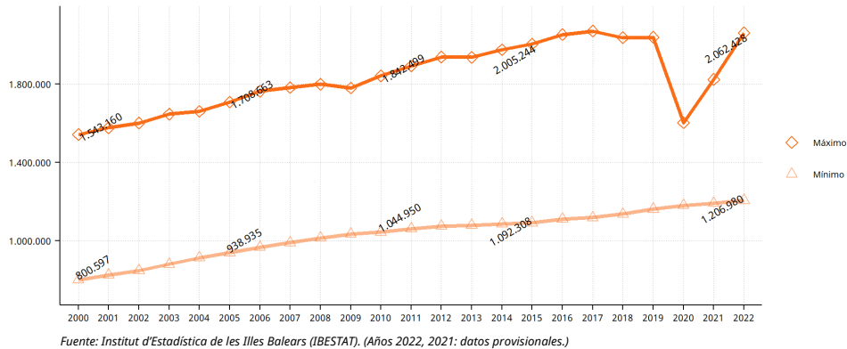
Valores máximos y mínimos anuales del indicador de presión humana en las Illes Balears: 2000-2022
